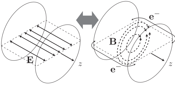
図 14: ピルボックス空洞内の電場 \mathbf{E} と磁場 \mathbf{B} 。時間的に電場と磁場が入れ替わる。 e^- は電子 (壁面電流) の動きを示したものの。
