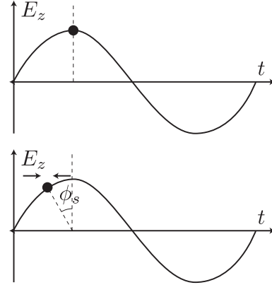
図 15: リニアックにおける同期位相。縦軸は加速ギャップ中央での電場振幅 E_z 、横軸は時間 t 。(上) 電子リニアックの場合。速度はほぼ光速に近いので位相振動がなく。振幅最大となる位相 \phi = 0 を用いる。(下) 陽子リニアックの場合。電場が時間的に増加する側では、時間的に早い粒子は受ける電場が小さいため遅れ、一方、時間的に遅れてきた粒子は平衡点にある粒子よりも加速されるため、結果的に平衡点に近づく。
