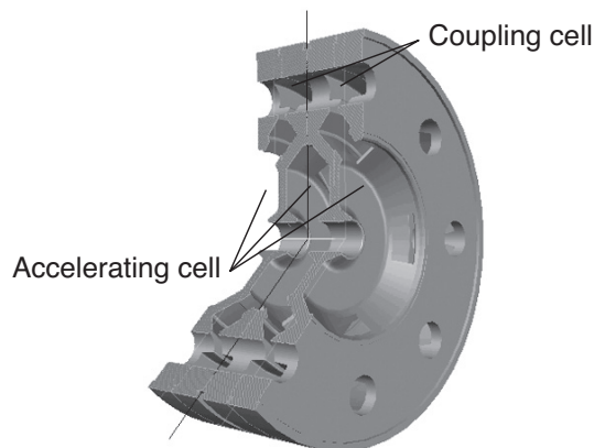
図 35: Annular-ring coupled structure (ACS) 型加速管。結合セルをビーム軸まわりにリング状にし、ビーム軸周りの電場の軸対称性を上させたもの。
