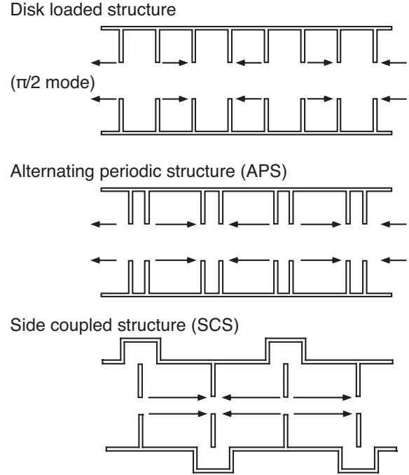
図 33: \pi/2 モード加速管の発展。(上) ディスクロード型を \pi/2 モードで励振した場合の電場分布。(中) APS 型加速管。 \pi/2 モードで励起されないセルを短くしてシャントインピーダンスを高めた。(下) サイドカップル型加速管。 \pi/2 モードで励振されないセルをビーム軸上からずらして外側に配置したもの (図 34 に立体図を示す)。同様の構造に Disk-and-washer (DAW) 型加速管や Annular-ring coupled structure (ACS) 型加速管がある。
