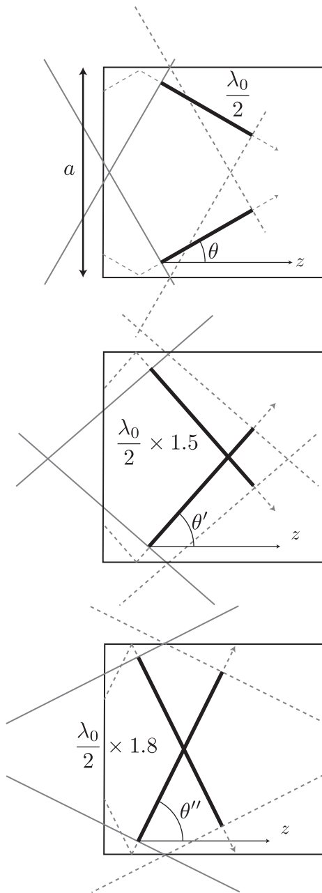
図 19: 自由空間での波長 \lambda_0 が長くなると、 z 方向と角度 \theta が大きくなる。波長の上限 \lambda_c を遮断波長といい、導波管の長辺方向の長さ a と a = \lambda_c/2 なる関係をもつ。
