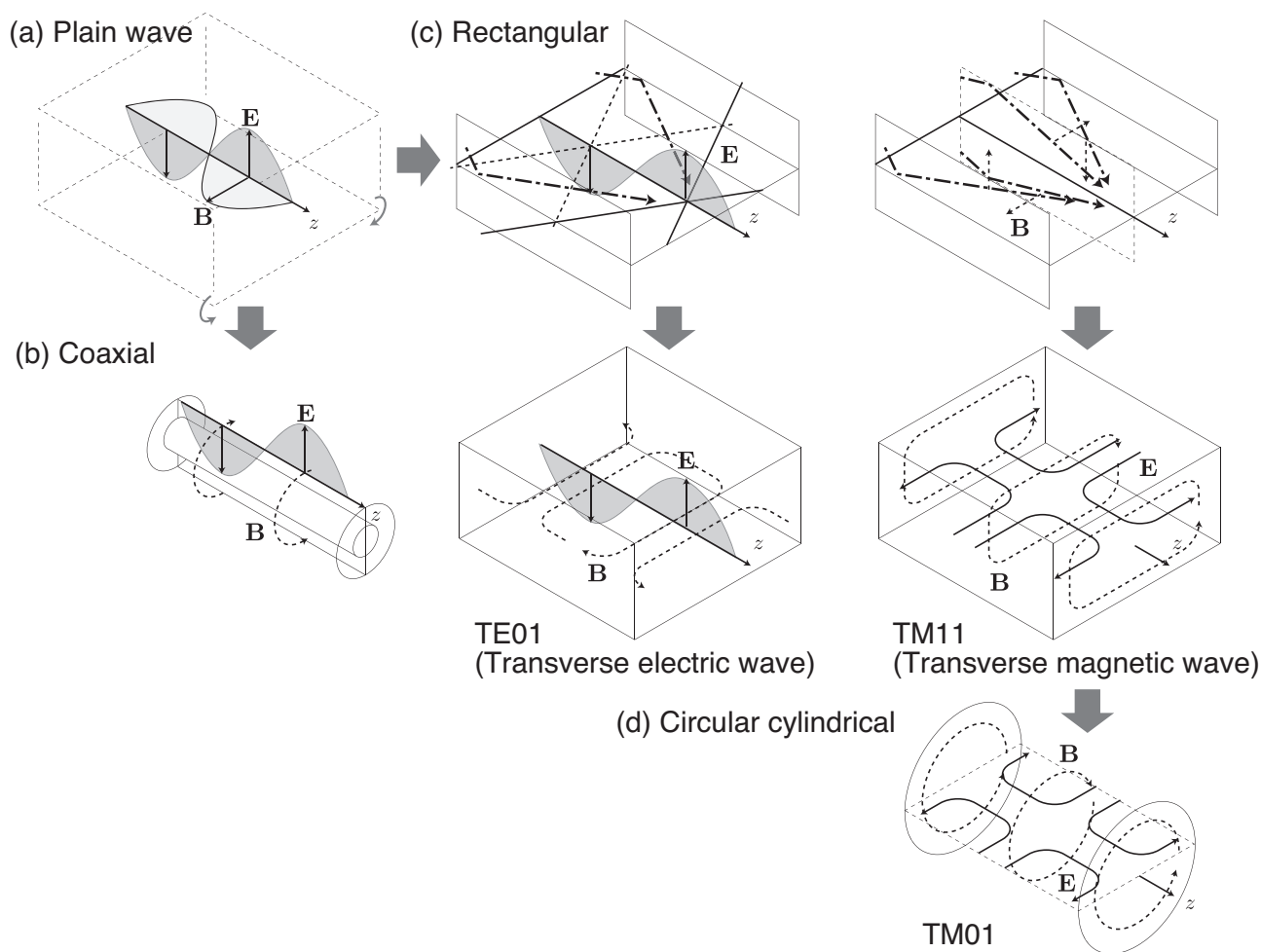
図 13: 同軸管、方形導波管、円形導波管中の電磁場。作図では導波管の外形の一部を表す点線を除き、実線は \mathbf{E} 、点線は \mathbf{B} 、一点鎖線は \mathbf{S} を示す。(a) 平面波の上下 ( E 面) に導体を設置しても電磁場の様子に変化はない。(b) 上下の導体をぐるっと巻くと同軸管になる (TEM 波)。(c) 左右の面を導体で覆うと、左右の面に沿って \mathbf{E} = 0 となる境界条件を満たすため平面波は斜行して反射しながら進む。左右の壁から反射された平面波が重ね合わさった結果、磁場は破線で示すように渦を巻く (TE 波となる)。同様に上下左右の壁で反射して磁場が進行方向に対して直角となる成分しか持たない場合は TM 波となる (同様に TE 波も成立可能で縮退している)。(d) 方形導波管の TM11 モードを円形導波管に変形すると、加速空洞で用いられる TM01 モードと考えることが出来る。いずれも導波管の中では平面波が壁面を反射しながら進んでいる (注: 上図で (a) の平面波の波長に対して TE01 は正しく作図したが、TM11, TM01 の管内波長は正しくない。電磁場のパターンのみを参照されたい)。これら導波管の中を進んでいく電磁場は進行波と呼ばれる。
