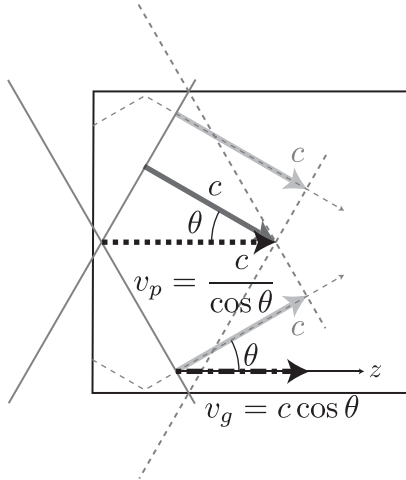
図 17: 導波管内の位相速度 v_p と群速度 v_g 。もとなる二つの波が光速 c で進むとき、見かけ上の速度は v_p > c となることがわかる。
