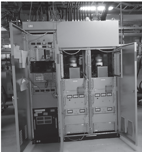
Fig. 33 FC 用パルス電源の外観。
