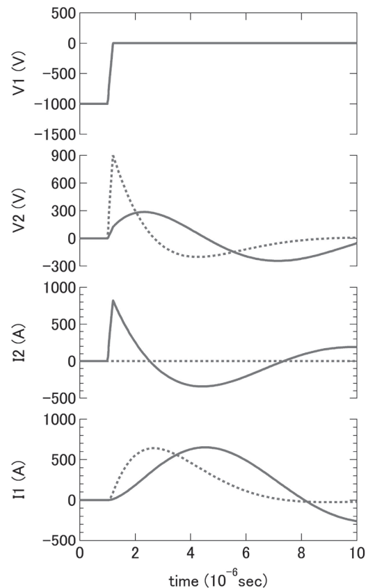
Fig. 36 LT Spice による Fig. 35 の回路の計算結果。 C1 = 2 \mu\text{F} (実線)、1 fF (実線)
