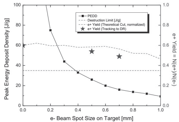
Fig. 16 ターゲット上のビームサイズ (直径) と PEDD のシミュレーション結果
