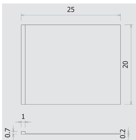
Fig. 32 スリットに挿入した ZrO_2 製 0.2 mm 厚のスペーサー。
