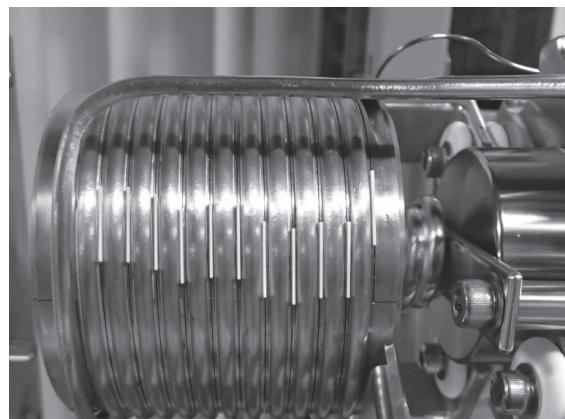
Fig. 31 スペーサーを挿入した状態の FC。
