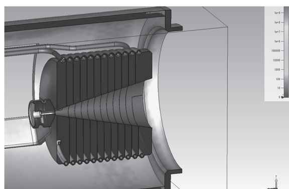
Fig. 19 FC にパルス電流を流した際の発熱分のシミュレーション結果。
