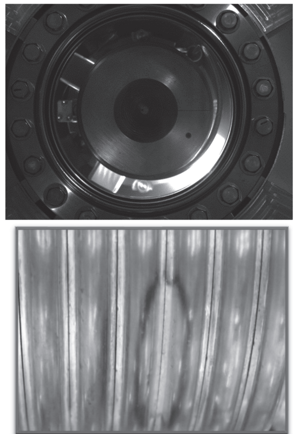
Fig. 23 放電時の様子を下流からビューポート越しに撮影した写真 (上)。大きな放電が発生した痕跡 (下)。
