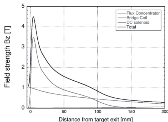
Fig. 11 ターゲット付近のビーム軸方向磁場強度[13]。
