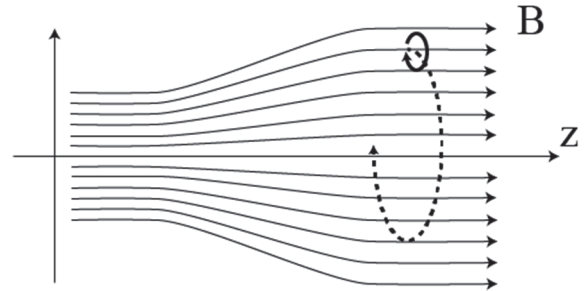
Fig. 6 ミラー磁場と其中での荷電粒子の軌道
