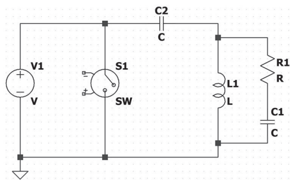
Fig. 34 FC 用パルス電源の動作原理を示す回路図。
