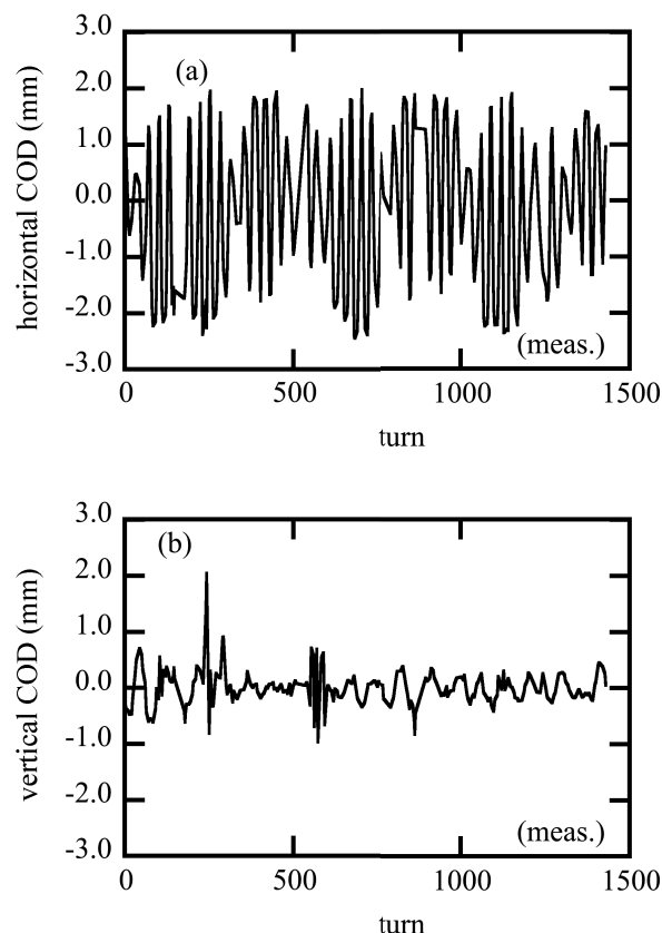
Fig. 2 補正前の(a) x 方向及び(b) y 方向の COD @ BPM.
