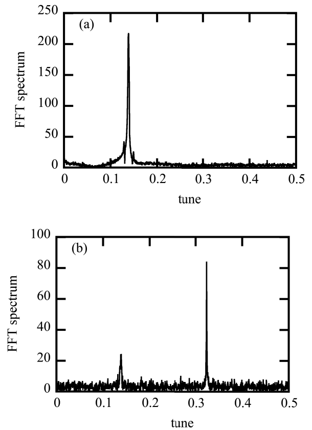
Fig. 6 Fig.4 について 1000 ターン分のデータをフーリエ級数展開したもの。横軸の 1 ステップの刻みを「サンプリングターンの逆数（今回は 1000 ターンサンプリングしたので、横軸の 1 ステップは 0.001）」としてグラフを描けば上手になる。
