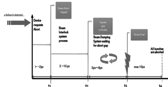
Fig.8 アボートトリガー所要時間
