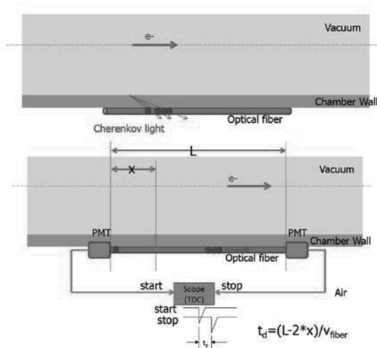
Fig.4 光ファイバーの原理[3]
