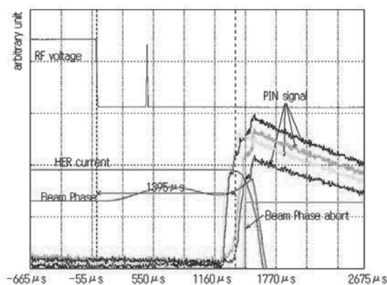
Fig. 16 コリメータが傷ついた時のアボート例
