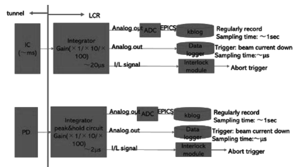
Fig.14 ビームロスモニター信号の流れ
