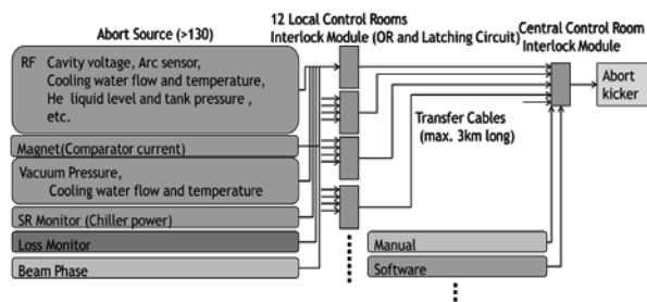
Fig.7 アボートトリガー信号
