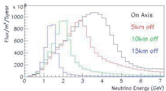
図 3：Off Axis ビーム
