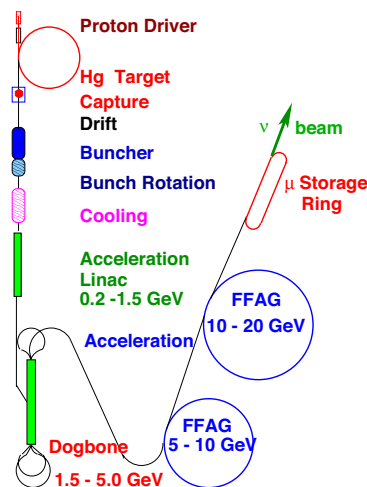
図 10: US ニュートリノファクトリの模式図 (Study IIA)
