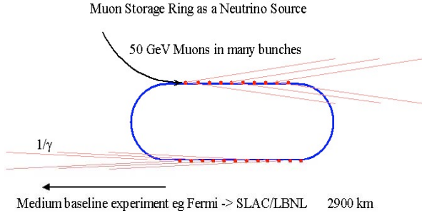
図 8: ミューオン貯蔵リングとニュートリノビームの広がり
