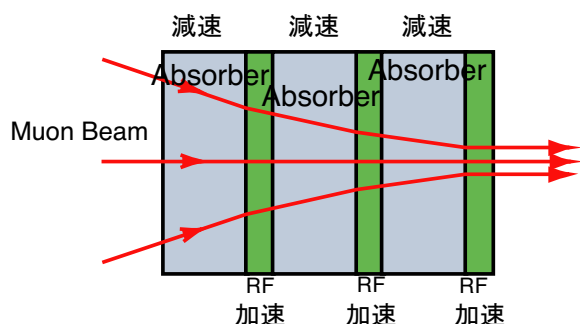
図 7：イオン化冷却の原理
