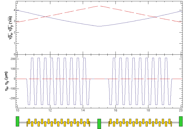
図 14: TESLA のウイグラー (1 セル)。
