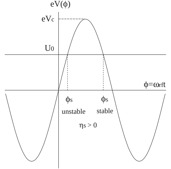
図1: 同期位相。遷移エネルギーよりも大きなエネルギー領域の場合。
