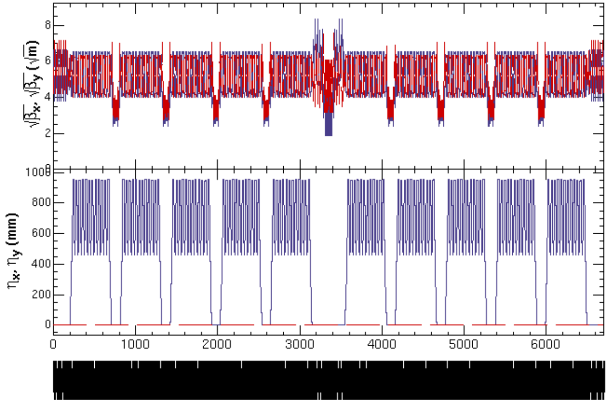
図 19: OCS ラティス。
