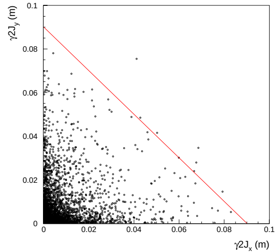
図 10: 陽電子入射ビームの規格化ベータトロン振幅 (シュミレーション)。
