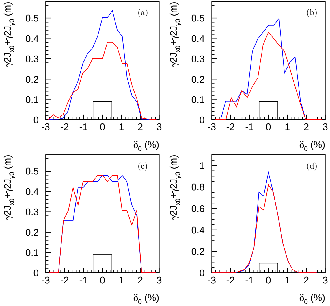
図 16: ダイナミック・アパーチャー。(a) TESLA dogbone、(b) MCH( V_c = 115 MV)、(c) OCS、(d) PPA。青色は磁場の誤差のない場合、赤色はマルチポール磁場の誤差を入れた場合。
