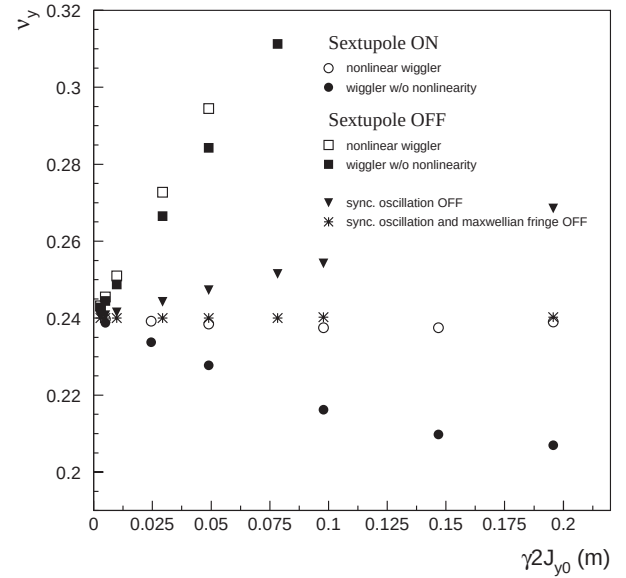
図 12: TESLA dogbone リングについての垂直方向のチューンの振幅依存。丸印は六極磁石をオン、四角印、三角印、バツ印はオフした場合。三角印はシンクロトロン振動をオフ。バツ印はシンクロトロン振動オフ、全ての磁石のマクスウェル・フリンジ磁場をオフ。
