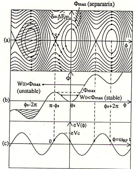
図 3: セパトリックス (separatrix)。
