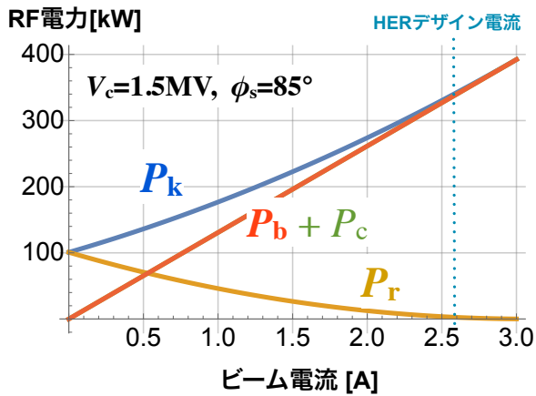
図 6.11 optimum tuning & optimum coupling 条件において超伝導空洞 ( \phi_s = 85^\circ ) で必要な RF パワー (SuperKEKB の HER 運転の例)。
