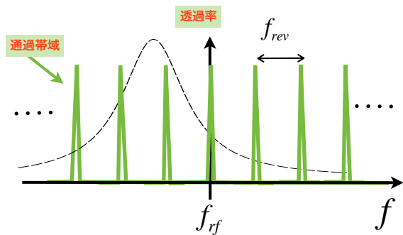
図 8.19 CBI ダンパ用 FB ループにおける楕形フィルタの透過特性
