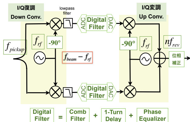
図 8.20 一般的な CBI ダンパのフィルタ構成
