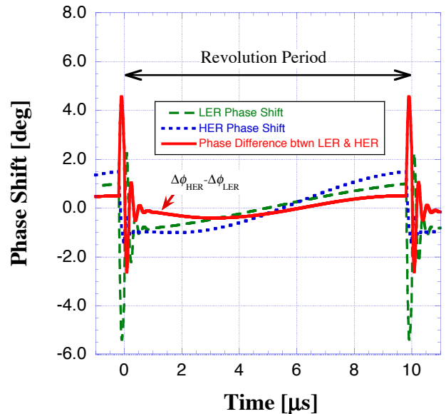
図 10.9 HER と LER の位相変化の相対的なズレ ( \Delta\phi_{\text{HER}} - \Delta\phi_{\text{LER}} )
