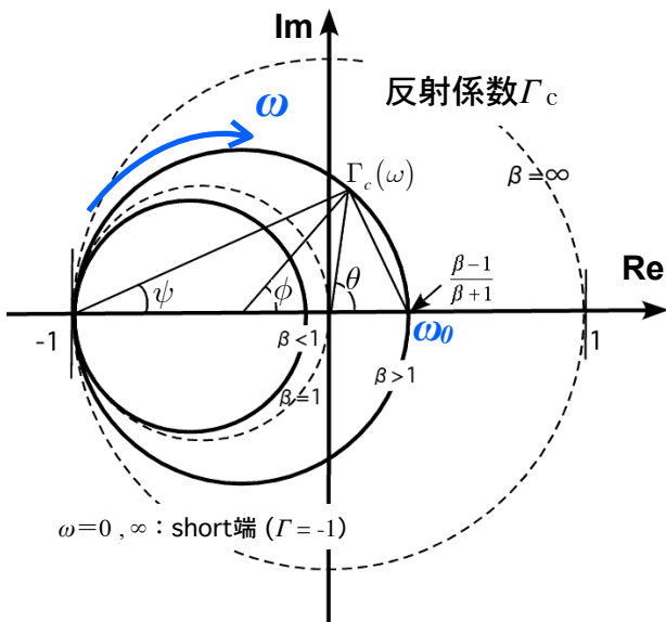
図 5.5 共振器の反射係数 \Gamma_c(\omega) の複素平面プロット ( \omega 変化による軌跡)
