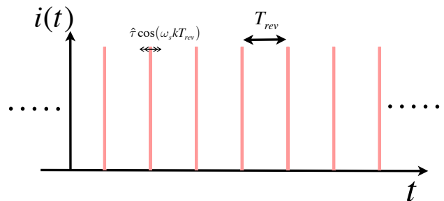
図 7.5 縦方向に微小振動するポイント・バンチ 1 つが周回している場合のビーム信号（時間領域）
