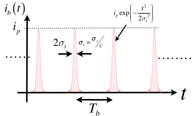
図 6.1 Gaussian バンチ・トレイン
