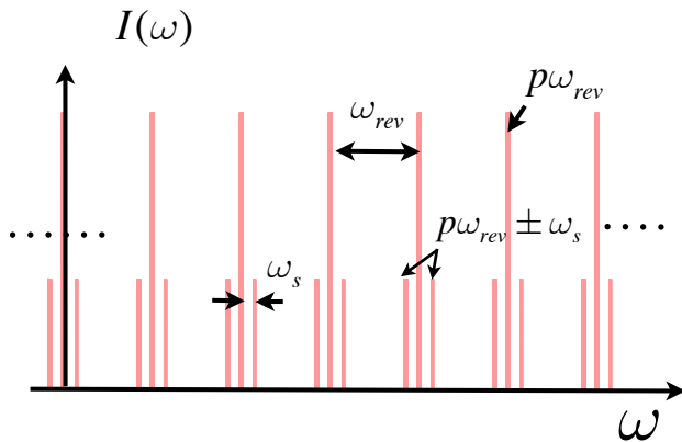
図 7.6 シンクロトロン振動周波数 \omega_s で振動しているポイント・バンチが 1 周回している場合の周波数スペクトル
