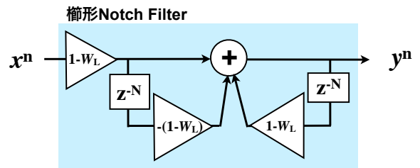
図 8.27 comb filter を逆特性にした楕形 notch filter のブロック図
