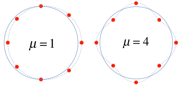
図 7.8 図 7.7 をリング上に示したもの ( h = 8, \mu = 1, 4 の場合)。図では、分かり易くするために横方向の変位で表している。
