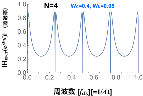
図 8.29 double peak comb filter の周波数特性 (伝達関数 |H_{\text{NF}}(e^{j\omega})| ) のプロット ( N = 4, W_C = 0.4, W_N = 0.05 の例)
