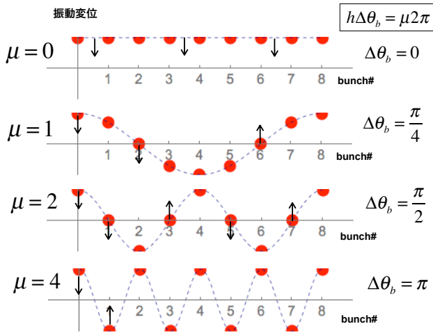
図 7.7 バンチ結合による振動モード ( h = 8, \mu = 0, 1, 2, 4 の場合)。 \mu はモード番号。縦軸は振動の変位、横軸はバンチ番号を表す。8 番目は元のバンチ (0 番目) と同じ。
