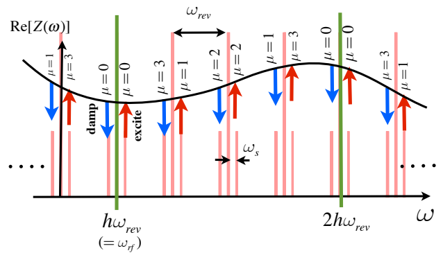
図 7.9 各振動モード \mu とインピーダンス (excite, damp) の関係。 h = 4 の場合の例。式 (7.37) で p = 1 の周りを示している。矢印の上向きが excite、下向きが damp を表す。
