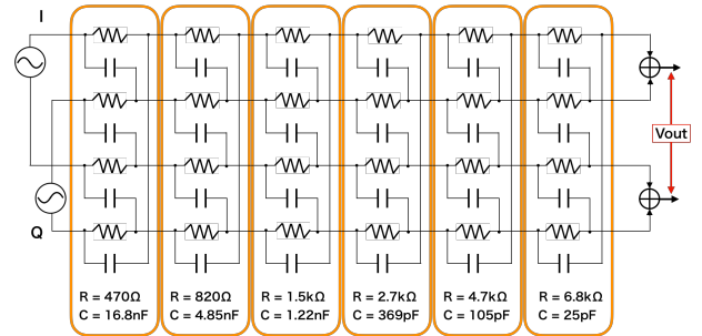
図 8.11 90° polyphase filter の回路図
