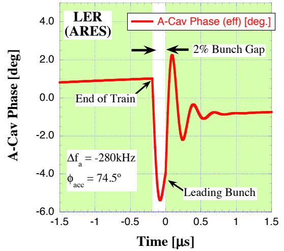
図 10.5 LER の ARES 空洞における BGT による位相変調（ギャップ前後を拡大）
