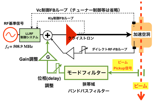
図 8.1 結合バンチ不安定性を抑える FB ループ (CBI ダンパーシステム) のブロック図
