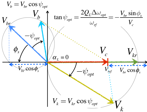
図 6.8 \alpha_L = 0 になるように最適に detuning し、 V_c = V_{ref} となった場合。
