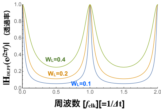
図 8.22 デジタル LPF の周波数特性 (伝達関数 |H_{DLPF}(e^{j\omega})| ) のプロット ( W_L = 0.1, 0.2, 0.4 の例)
