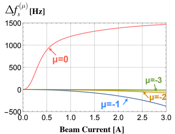
図 7.15 バンチ間結合に起因するシンクロトロン振動の周波数変化。SuperKEKB の HER デザインにおける計算値
