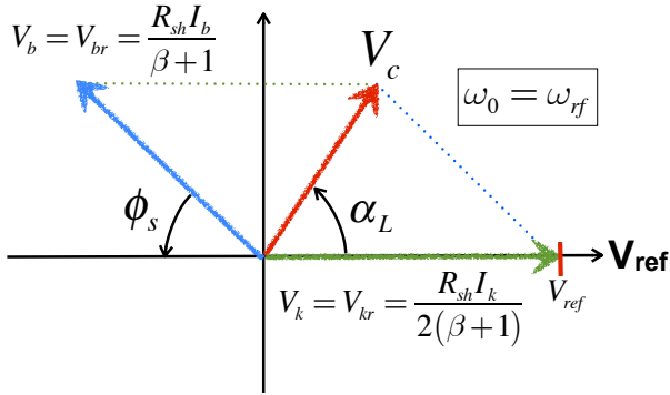
図 6.6 \omega_0 = \omega_{rf} において、RF 投入による電圧 V_{kr} とビーム励起電圧 V_{br} との合計。
