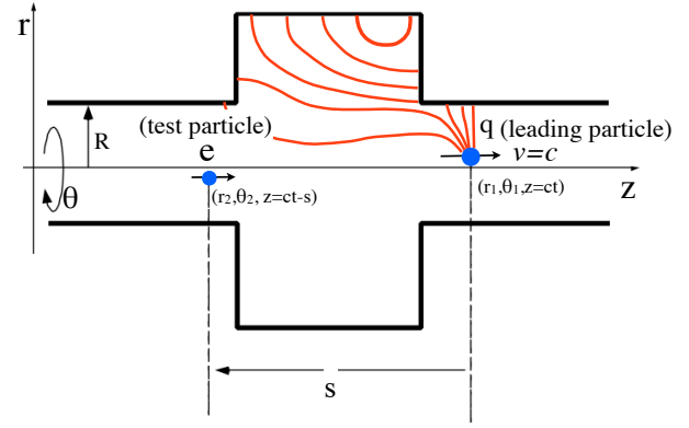
図 7.4 先行する点電荷 (leading particle) が励起した wakefield を後ろの電荷 (test particle) が感じる。
