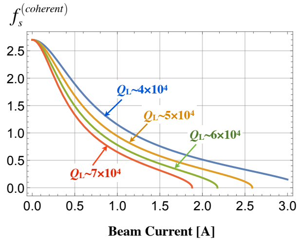
図 7.17 復元力が V_k だけの場合に、シンクロトロン振動周波数が下がる効果の評価 (HER の例)。
