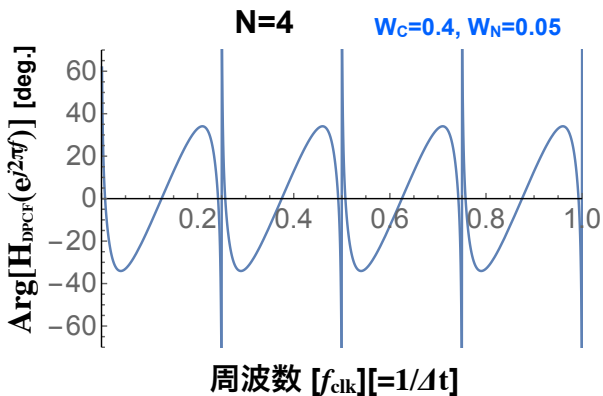
図 8.30 図 8.29 における伝達関数の位相特性
